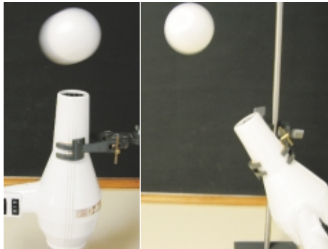
Figura 9: Bola flotante
